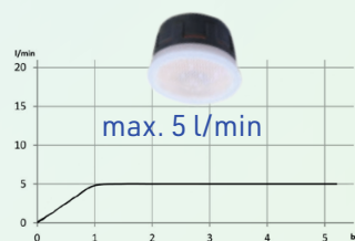
Vízátfolyás mosdókagyló betéttel
